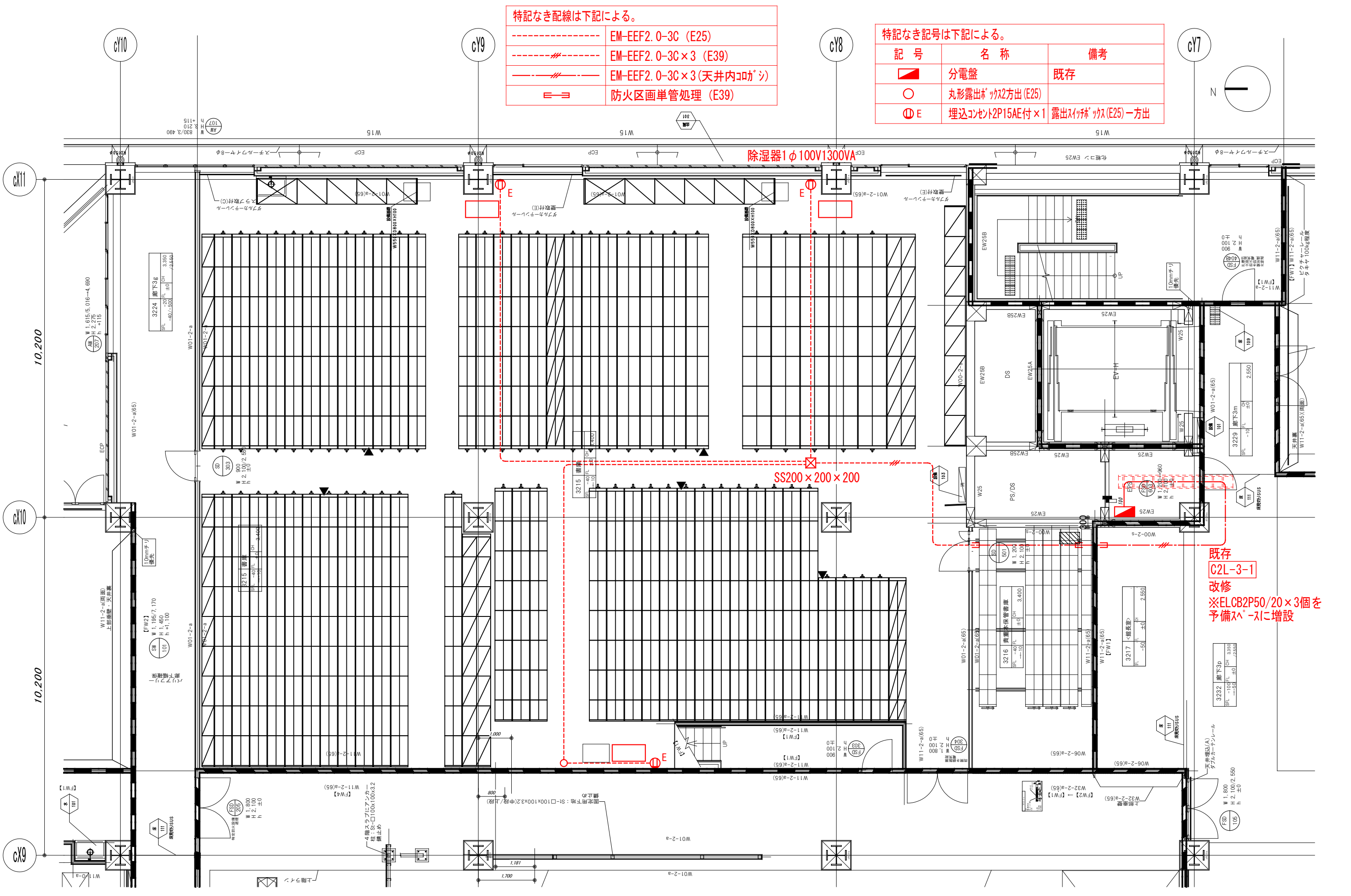
C棟3階書庫除湿器設置計画図 S=1/100 (A3)
