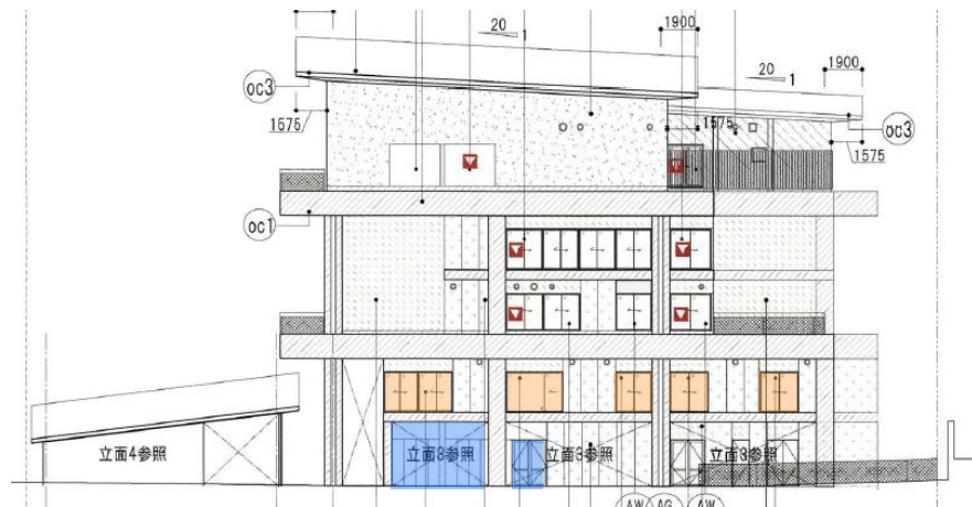
西側 立面図
