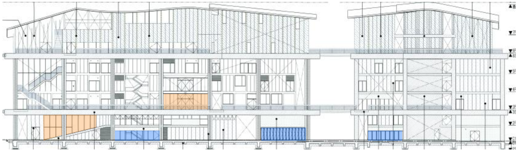
D棟
