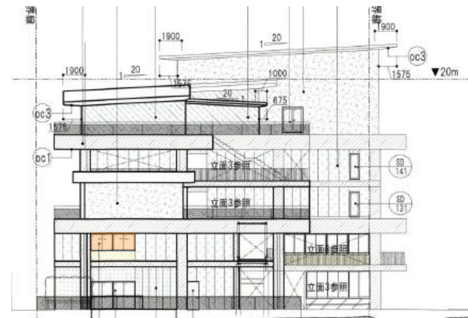
東側 立面図
