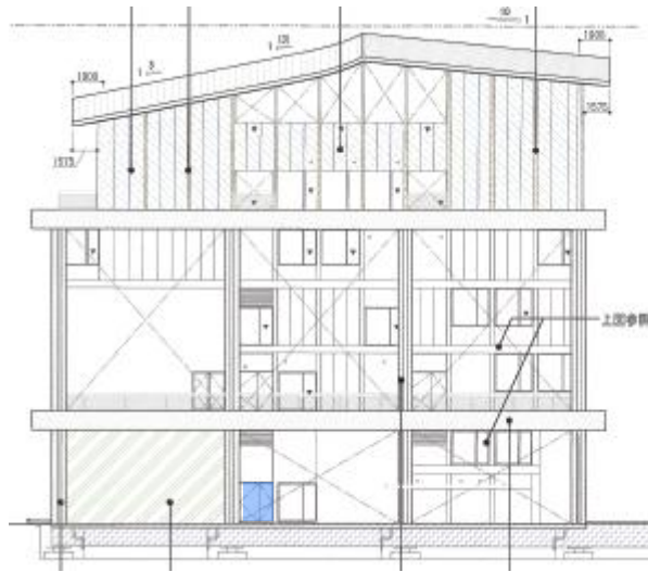
D棟
